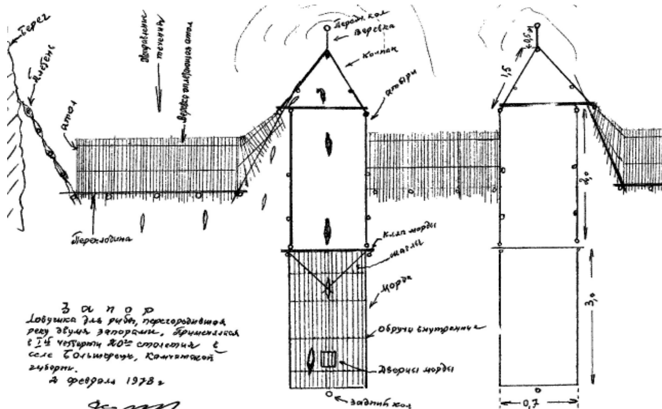
Устройство рыболовного запора (рисунок автора)
