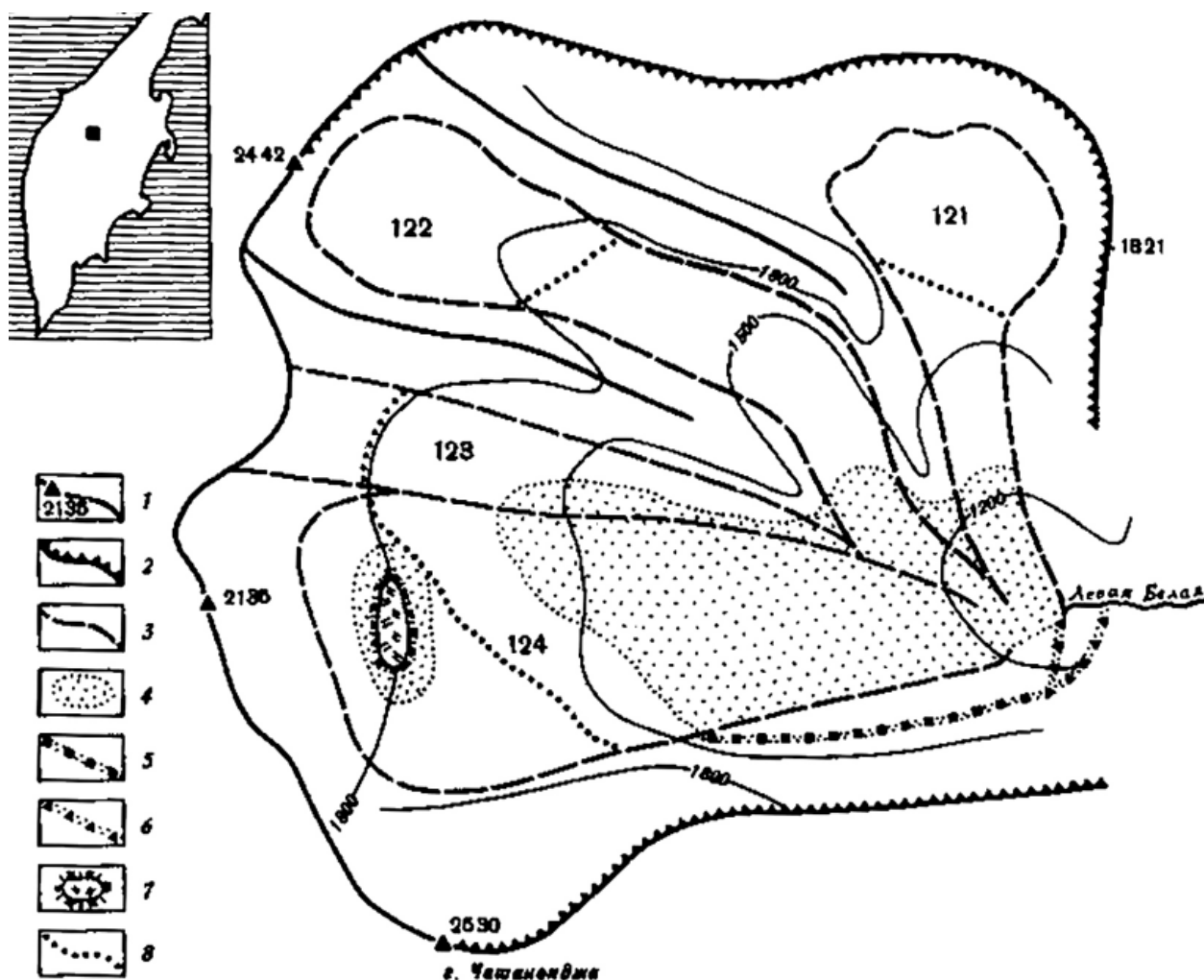
Схема ледников кальдеры вулкана Чашаконджа [4]:
